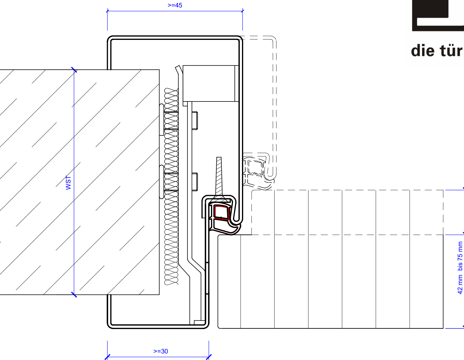
Stahlumfassungszarge zweiteilig Türblatt stumpf
