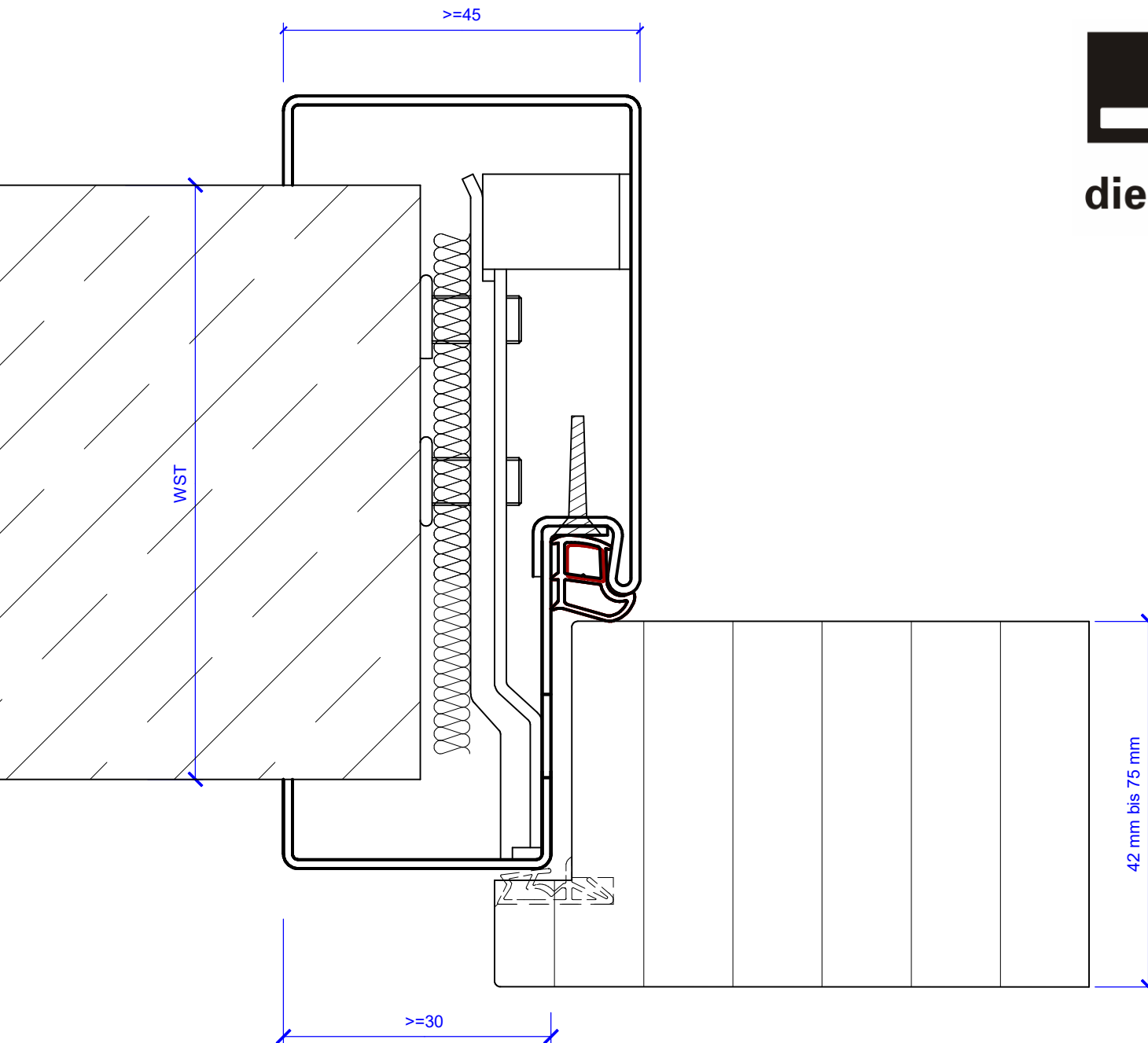
Stahlumfassungszarge zweiteilig Türblatt gefälzt
