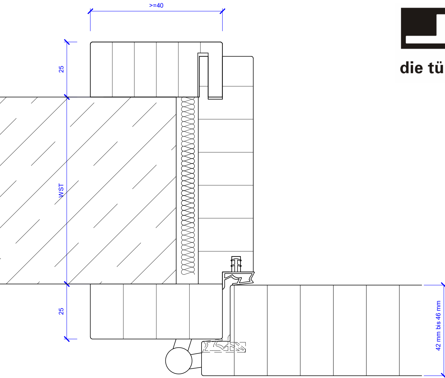
Holzumfassungszarge Türblatt gefälzt, 42-46 mm dick
