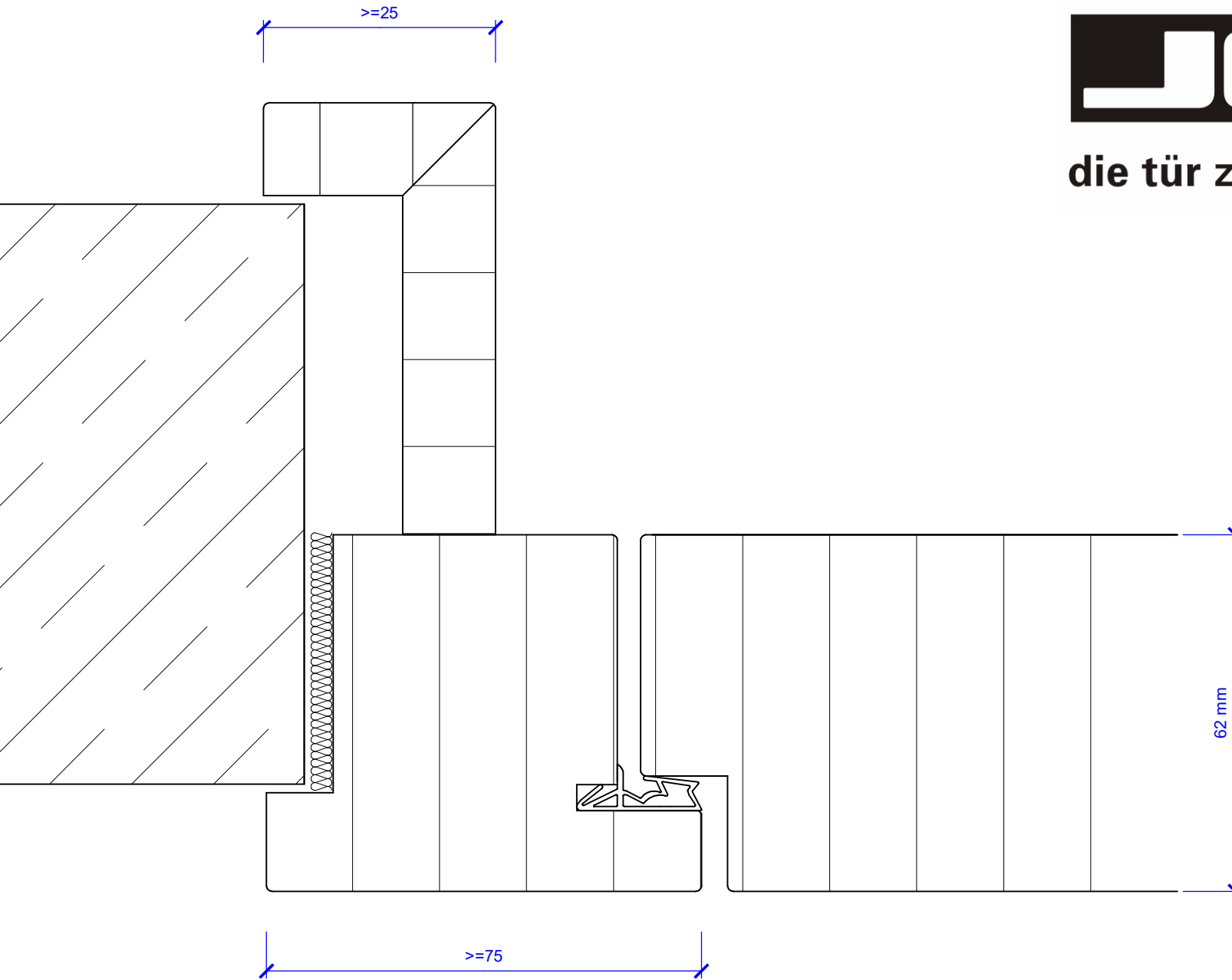
Holzstockzarge mit Gegenzarge Türblatt stumpf
